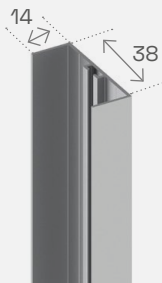
COMPENSATORE U-PROFILE COMPENSATEUR AUSGLEICHPROFIL
