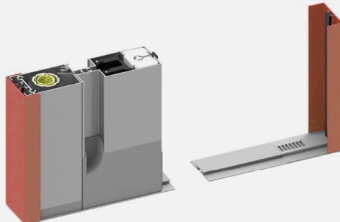
COMPENSATORE CASSONETTO E TERMINALE MAGNETICO ROLLER BOX U-PROFILE AND MAGNETIC U-PROFILE COMPENSATEUR BOÎTIER ET TERMINAL MAGNÉTIQUE AUSGLEICHPROFIL FÜR KASTEN UND MAGNETISCHES ENDPROFIL
